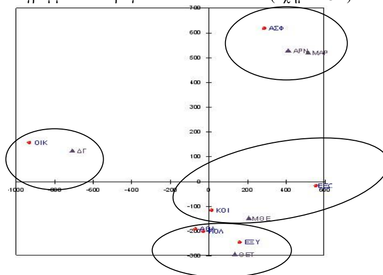
Σχήμα 13.1: Παραγοντικό επίπεδο 1x2 με ερμηνευτική ικανότητα 97,44%
